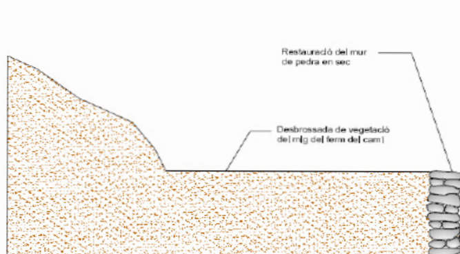
SECCIÓ TIPUS PROPOSDADA DEL CAMÍ
